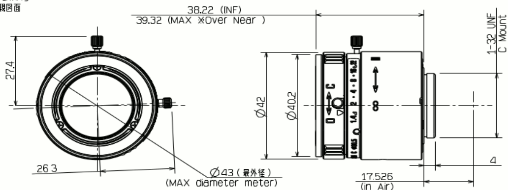
Drawing 外觀圖面
